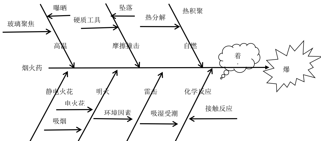
图 3.10-2 烟火药燃烧、爆炸触发条件分析图
