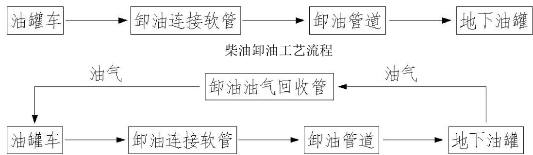
图 2-1 汽油卸油工艺流程
