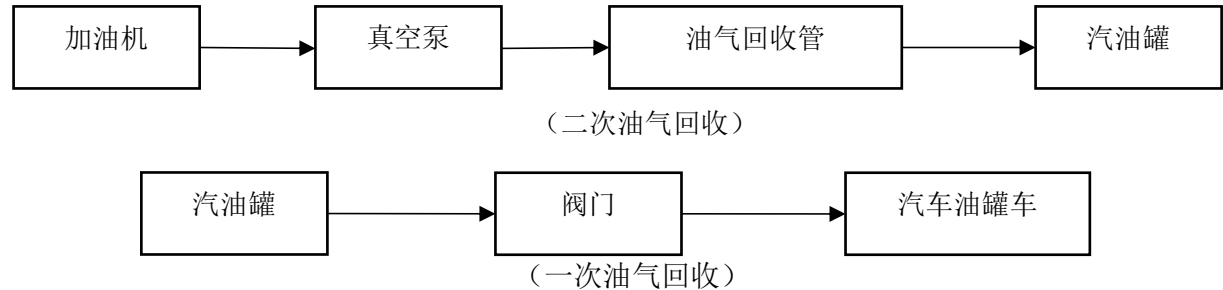
图 2-3 加油工艺流程简图
